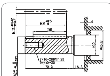
Albero - Shaft \varnothing 25,4 \text{ mm} Flangia - Flange Mod. K1
