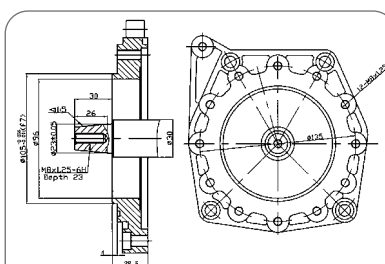
Albero - Shaft \varnothing 23 \text{ mm} Flangia - Flange Mod. FL "L"
