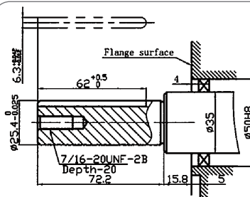
Albero - Shaft \varnothing 25,4 \text{ mm} Flangia - Flange Mod. K1
