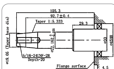
Albero - Shaft Mod. G1
