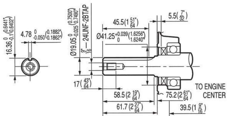
Albero - Shaft Mod.T/Q Ø 19,05 mm
