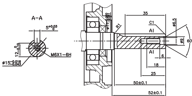
Albero - Shaft Mod.T/Q \phi 15 mm
