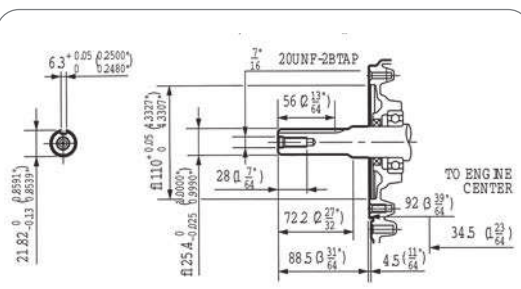
Albero - Shaft Mod.T/Q \varnothing 25,4 \text{ mm}
