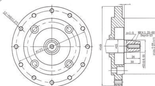
Albero - Shaft \varnothing 23 \text{ mm} Flangia - Flange Mod.FL "L"
