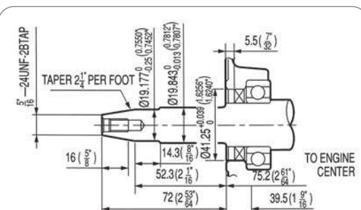
Albero - Shaft Mod.T/V
