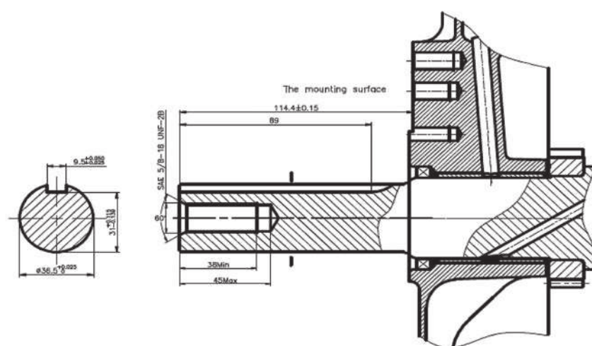
Albero - Shaft Mod.T/Q \varnothing 36,5 mm
