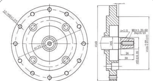
Albero - Shaft \varnothing 23 \text{ mm} Flangia - Flange Mod.FL "L"
