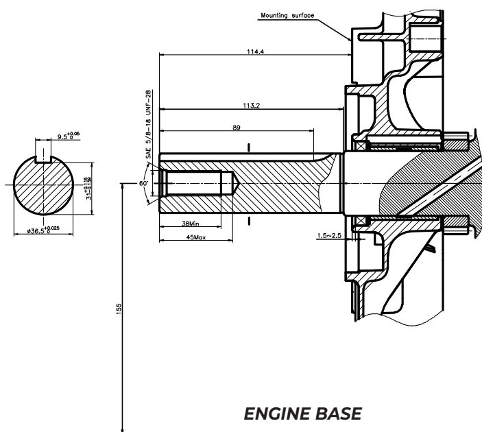
Albero - Shaft Mod.T/Q Ø 36,5 mm
