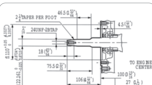
Albero - Shaft Mod.T/V
