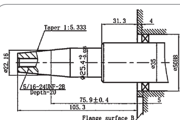
Albero - Shaft Mod. G1
