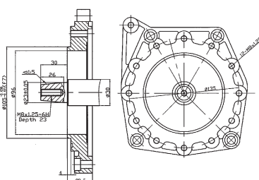
Albero - Shaft \varnothing 23 \text{ mm} Flangia - Flange Mod.FL "L"
