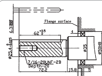
Albero - Shaft \varnothing 25,4 \text{ mm} Flangia - Flange Mod. K1
