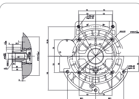
Albero - Shaft Ø 38 mm Flangia - Flange Mod.FL "L"
