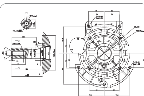
Albero - Shaft Ø 36,5 mm Flangia - Flange Mod. K1
